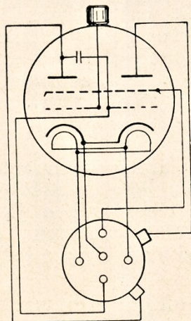
2HMD. Modulator-Doppelröhre (Oszillator und Modulator) für Superheterodyn-Empfang für Wechselstrombetrieb.
