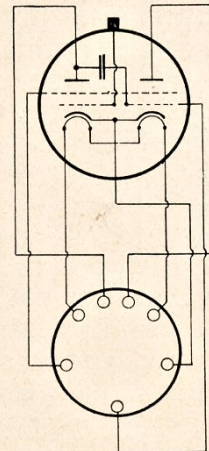
MO44. Modulator-Doppelröhre (Oszillator und Modulator) für Superheterodyn-Empfang für Gleichstrombetrieb.
