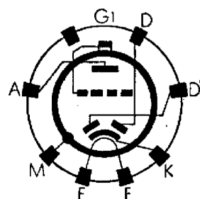
Sockelschaltung
